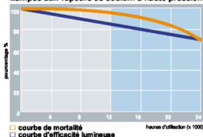
Lampes aux vapeurs de sodium à haute pression
